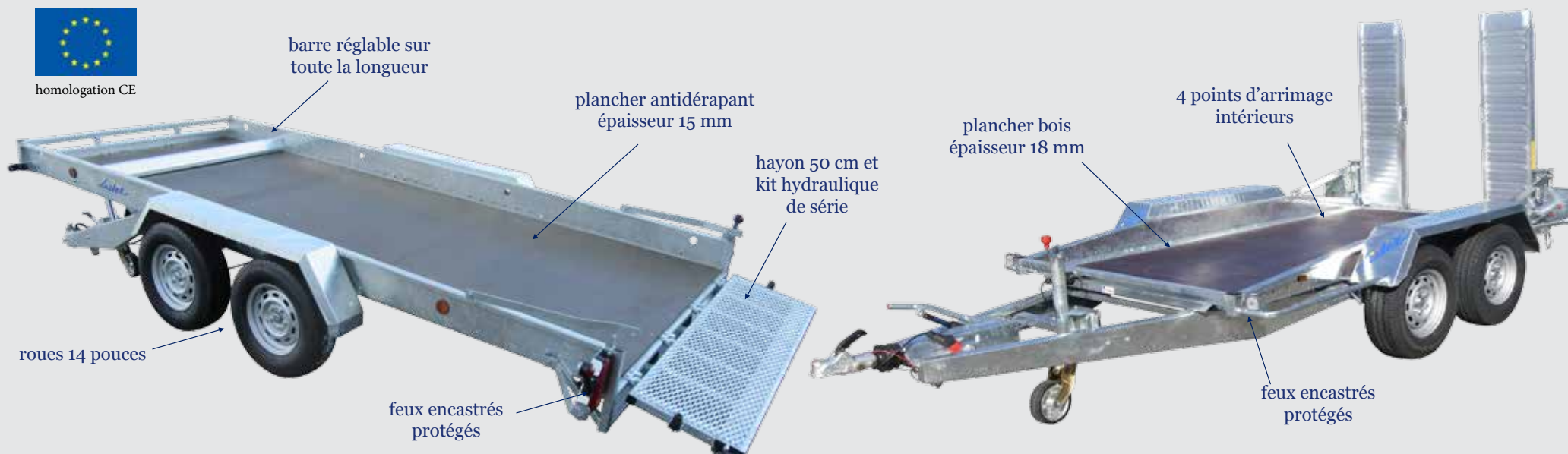
Modèle présenté : Porte-engin 35860
